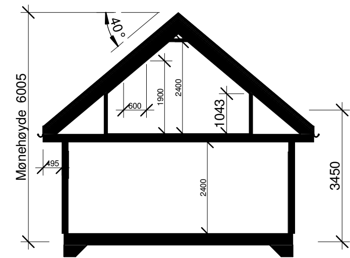
Snitt A - A
