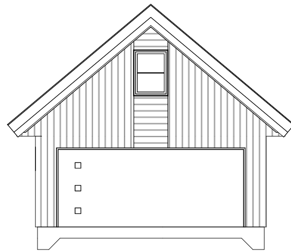
Fasade Øst
